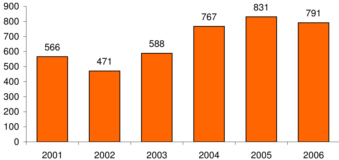
Anzahl der Niedrigenergiehäuser ≤50 kWh 2001 bis 2006
